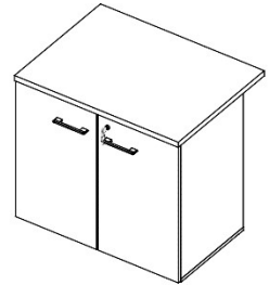
D25605 L800xA735xP450
