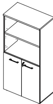
D25607 L800xA1630xP450
