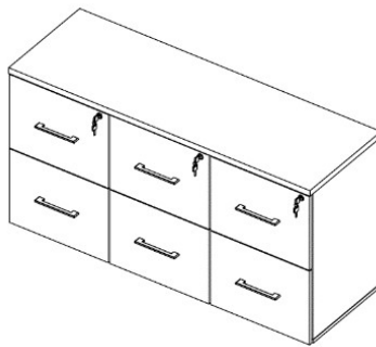
D25618 L1350xA735xP450
