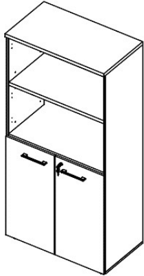
D25627 - L800xA1670xP450
