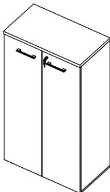
D25630 - L800xA1670xP450
