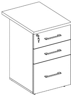
D25657 - L450xA735xP450/600
