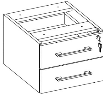
D25652 - L350xA260xP375
