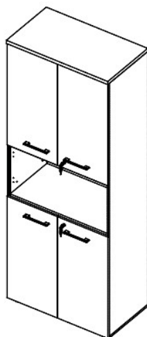
D25632 - L800xA2070xP450
