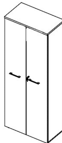
D25636 - L800xA2070xP450
