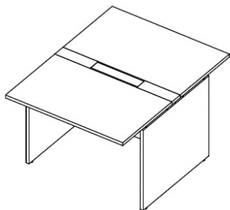
D25202 medidas L1000xA735xP1300 D25204 medidas L1200xA735xP1300 D25205 medidas L1400xA735xP1300
