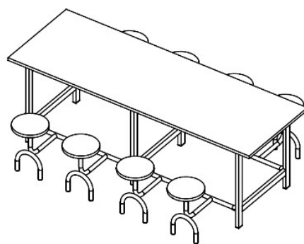
D25589 - L2400xA775xP800/1500
