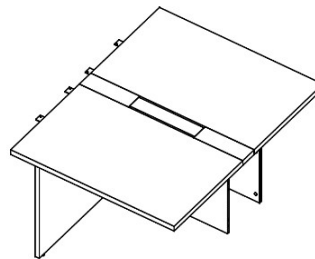
D25212 medidas L1000xA735xP1300 D25214 medidas L1200xA735xP1300 D25215 medidas L1400xA735xP1300
